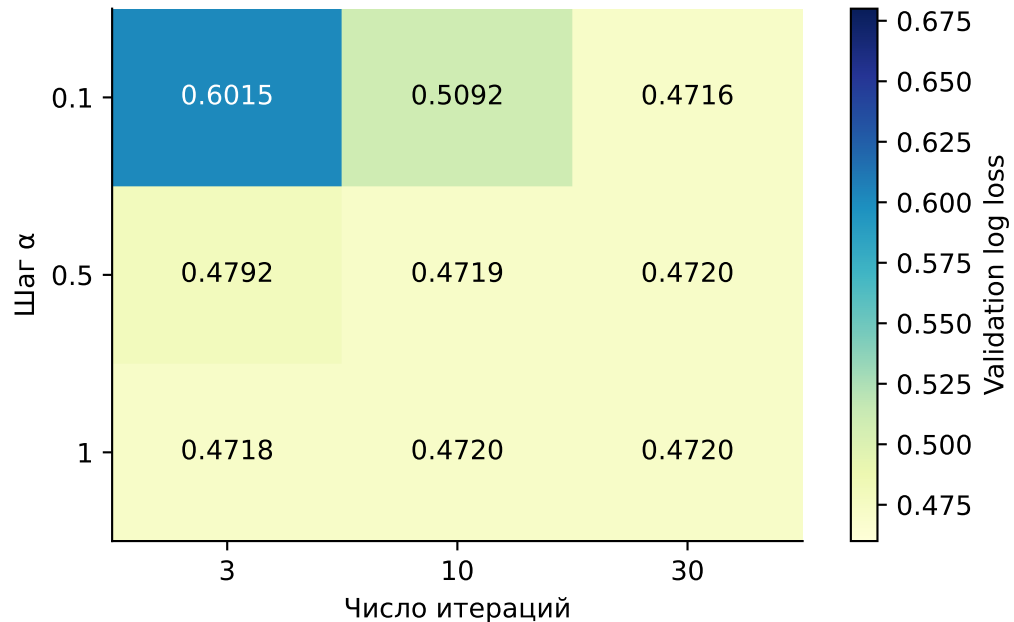
Метод Ньютона
