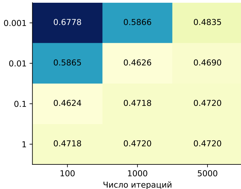
Градиентный спуск
